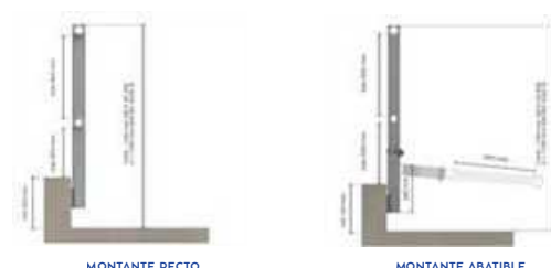
MONTANTE RECTO
